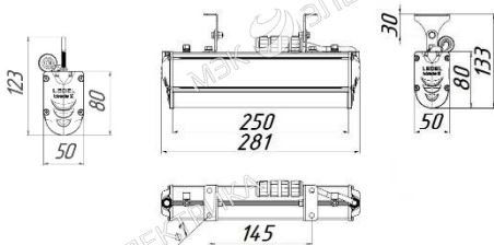
Рисунок 1 Светильник «L-trade II 12» подвесное крепление
