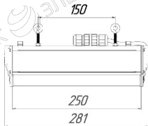
Рисунок 1 Светильник «L-trade II 12» подвесное крепление
