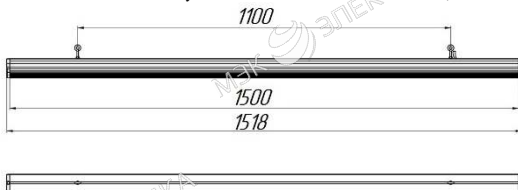
Рисунок 2 Светильник «L-fusion Office» 1,5 м
