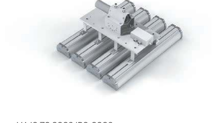
V4-IO-70.0003.IR0-0002 Консольное крепление для 4 светильников Размер крепления 465x220x276мм Установка на консоль диаметром 40÷50мм
