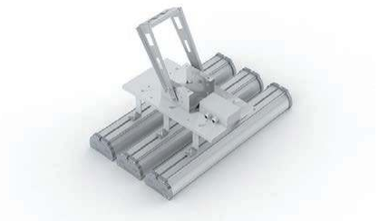
V4-IO-70.0002.IR0-0002 Поворотное крепление для 3 светильников Размер крепления 385x362x276мм (при положении скобы перпендикулярно светильникам) Угол поворота 180°, шаг 15°
