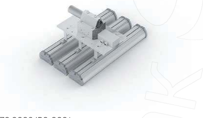
V4-IO-70.0003.IR0-0001 Консольное крепление для 3 светильников Размер крепления 385x220x276мм Установка на консоль диаметром 40÷50мм
