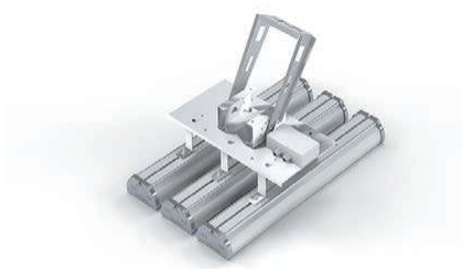
Возможность разворота скобы на 90° для удобства монтажа
