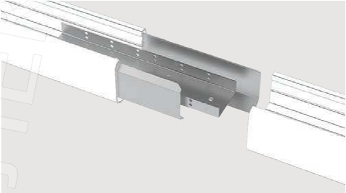
Комплект для соединения в линию Артикул: V4-R0-00.0009.Мм0-0001
