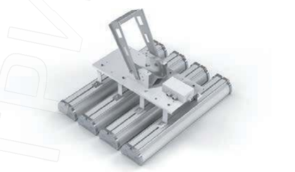
V4-IO-70.0002.IR0-0003 Поворотное крепление для 4 светильников Размер крепления 465x362x276мм (при положении скобы перпендикулярно светильникам) Угол поворота 180°, шаг 15°
