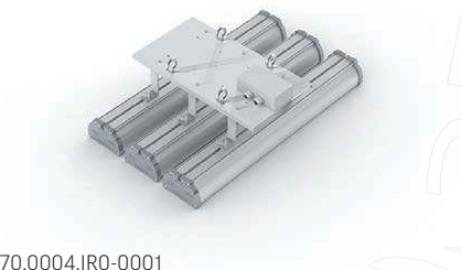
V4-IO-70.0004.IR0-0001 Подвесное крепление для 3 светильников Размер крепления 385x123x276мм
