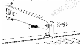
Рисунок 3 Установка светильника
