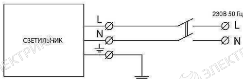
Рисунок 4 Схема подключения светильника
