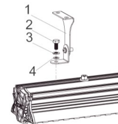
Рисунок 4 Монтаж крепления
