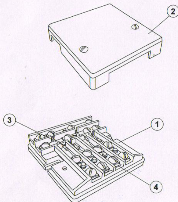
Рис.1 КОРОБКА РОН
